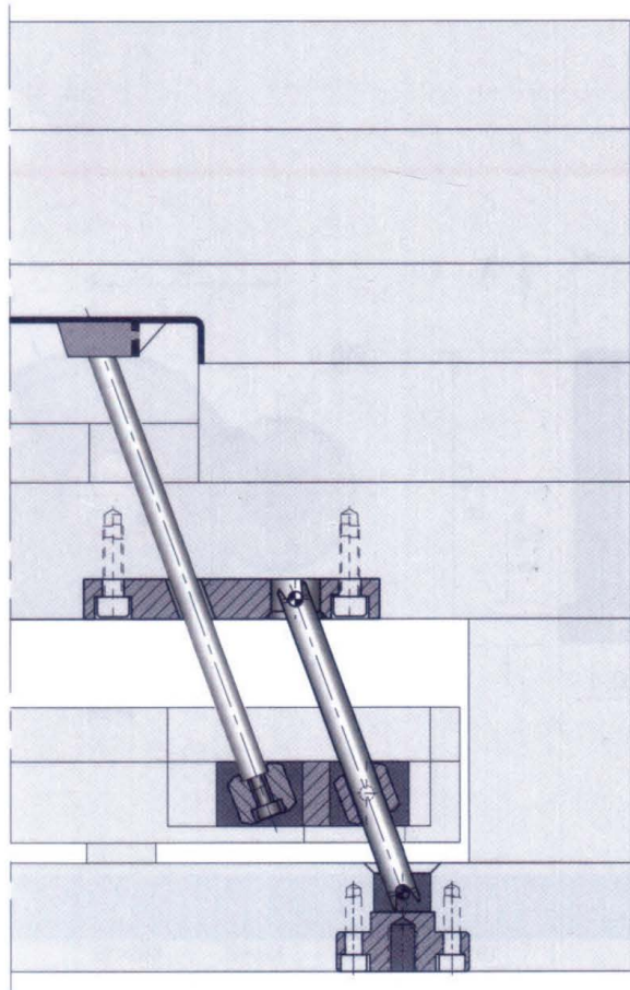
图1:合模状态
