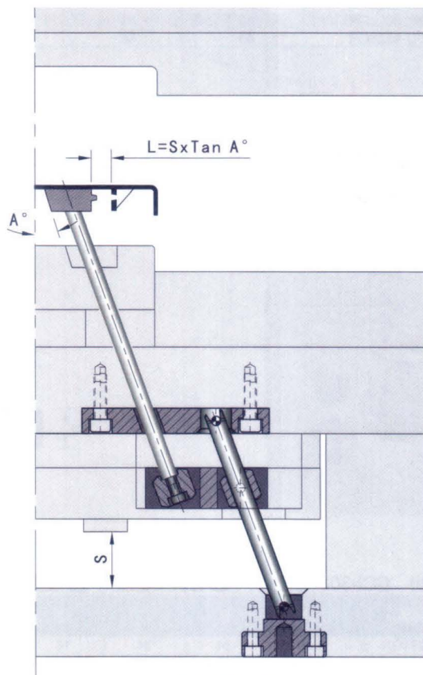
图2:顶出状态
